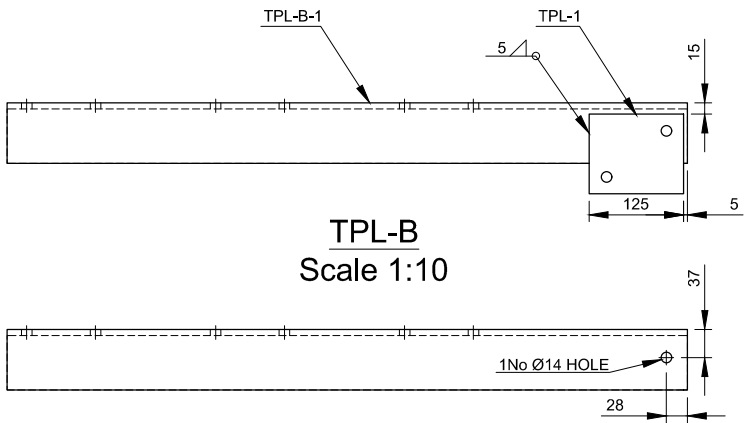
TPL-B-1 - EA 80x80x8 Scale 1:10
