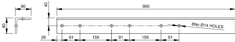
TPL-B-1 - EA 80x80x8 Scale 1:10
